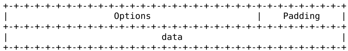
TCP Header Format
